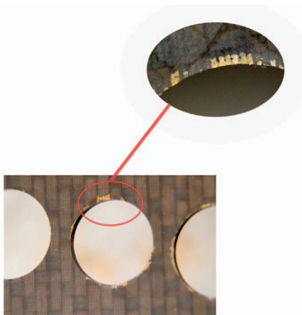
Bohrbearbeitung herkömmlich
