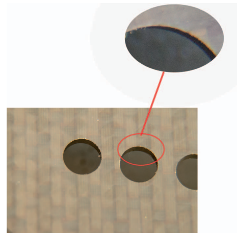
Bohrbearbeitung mit dem Bohrer C4600
